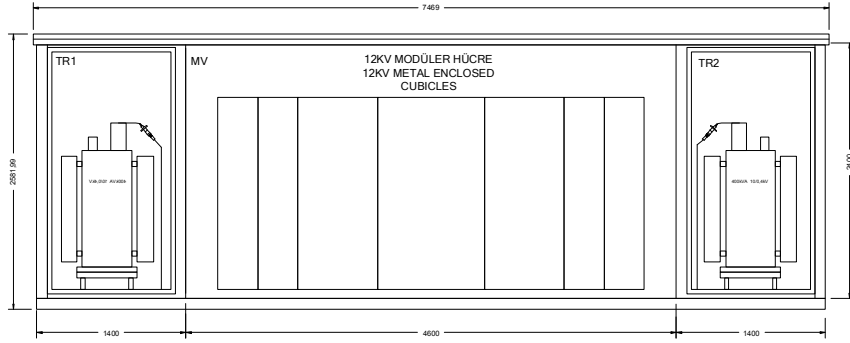
A GÖRÜNÜŞÜ A VIEW
